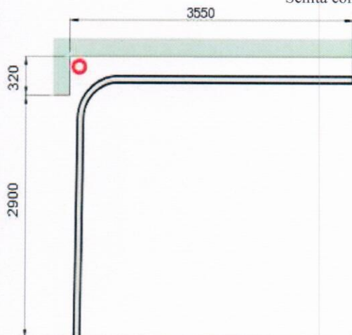
Schita confectie metalica
