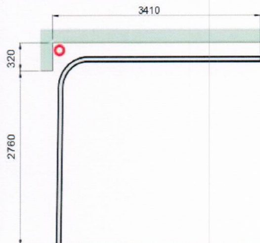
Schita confectie metalica
