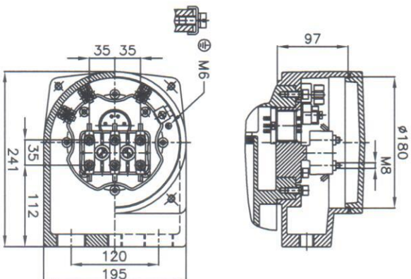
PRIKLJUČNA OMARICA Exe/TERMINAL BOX Exe
