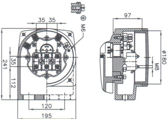
PRIKLJUČNA OMARICA Exd/TERMINAL BOX Exd
